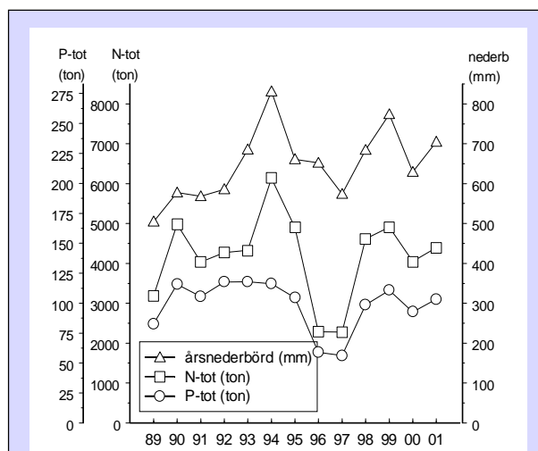
Nederbörd i Hanöbuktens avrinningsområde samt beräknad vattendragstransport av kväve och fosfor till kusten från de sex största vattendragen (Helgeå, Skräbeån, Mörrumsån, Bräkneån, Ronnebyån och Lyckebyån) 1989-2001.
