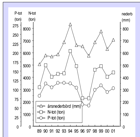
Figur 31 Nederbörd i Hanöbukstens avrinningsområde samt beräknad vattendrags-transport av kväve och fosfor till kusten från de sex största vattendragen (Helgeå, Skräbeån, Mörrumsån, Bräkneån, Ronnebyån och Lyckebyån) 1989-2001.
